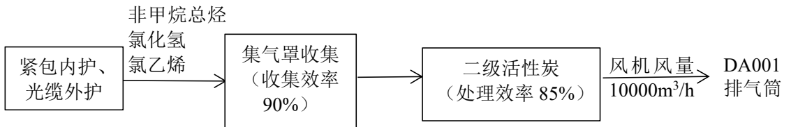
图4-1 废气收集及处理措施图
