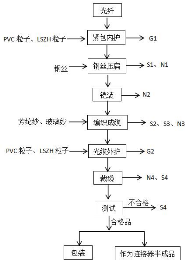
图 2-2 光缆制造工艺图
