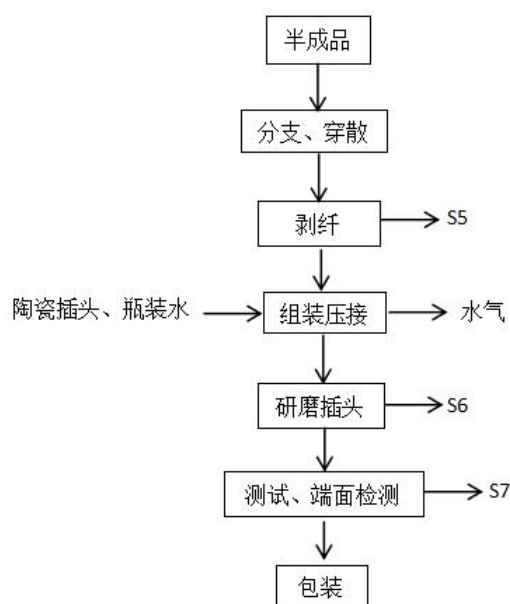
图 2-3 连接器制造工艺流程图
